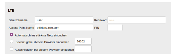
(Abb. 5: APN Einstellungen)
