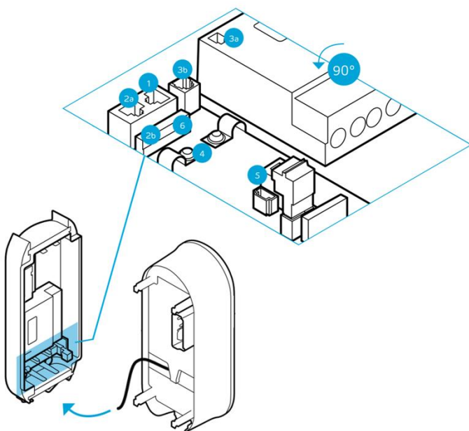
(Abb. 1: Übersicht Ports eBOX)
