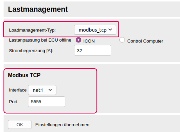
(Abb. 8: Modbus aktivieren)
